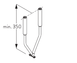
SG 6530 V-Hanger
